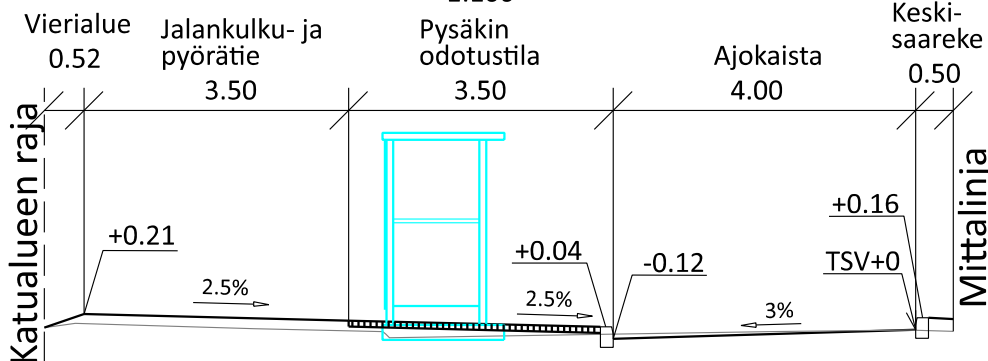
Tyypipoikkileikkaus A-A
