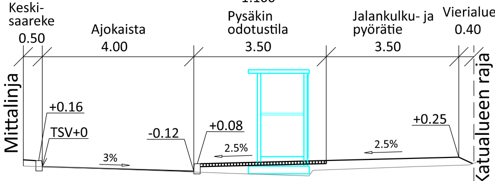
Tyypipoikkileikkaus B-B
