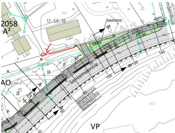
Kuva 2. Santamäentie XX etupihan hulevesien valumissuunta.
