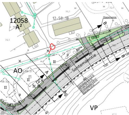
Kuva 1. Kartasta puuttuva viemäriyhteys
